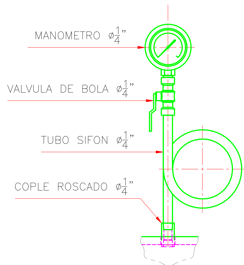
DETALLE DE CONEXION N1 ESC. 1:5
