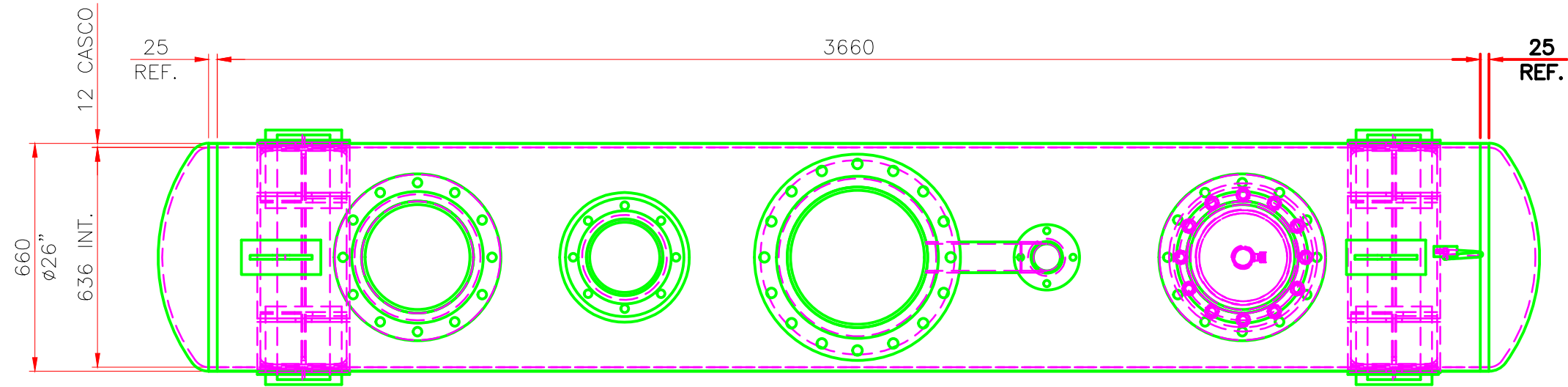
VISTA DE PLANTA ESC. 1:16
