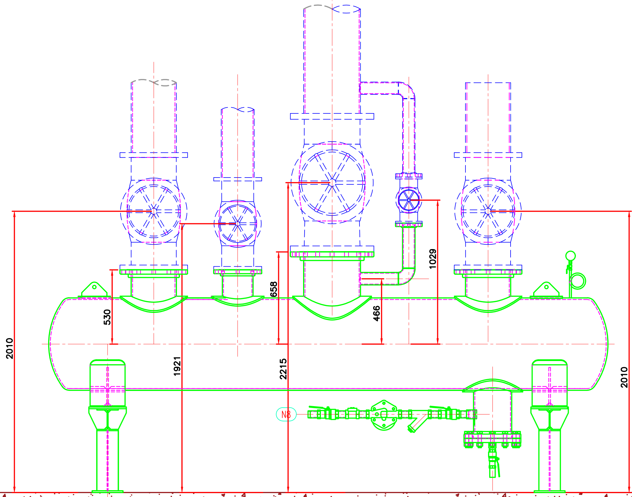
VISTA FRONTAL ESC. 1:16
