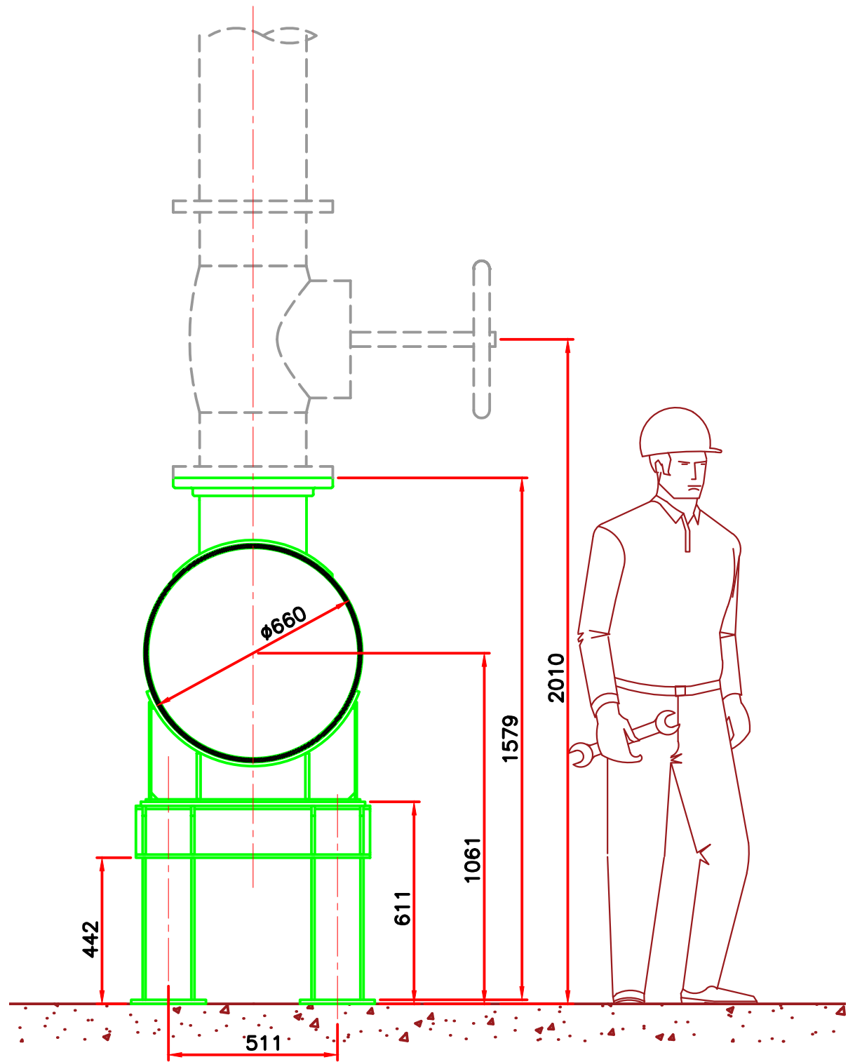
VISTA A-A ESC. 1:16
